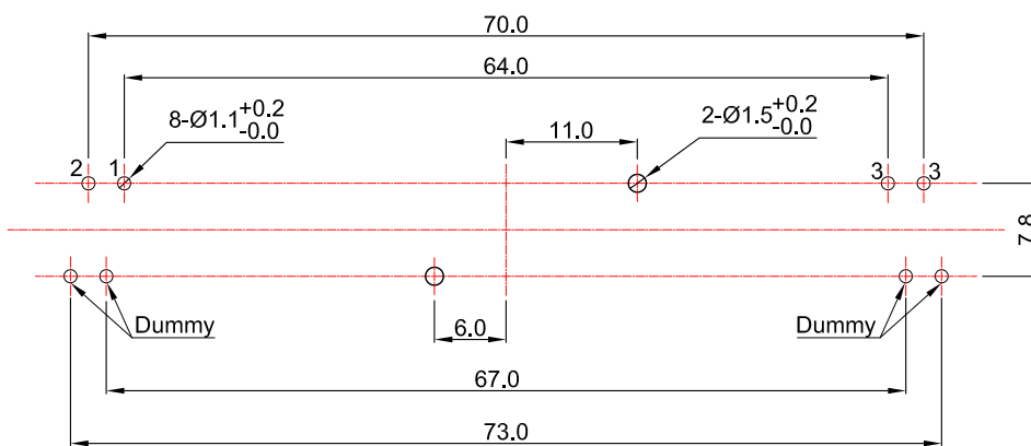
安装孔位图 P.C.B. mounting hole detail
