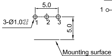
安装孔位置图 P.C.B. mounting hole detail
