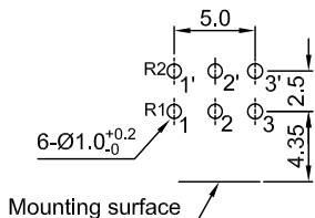
安装孔位置图 P.C.B. mounting hole detail
