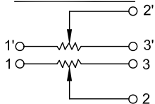
接线图 Circuit explanation
