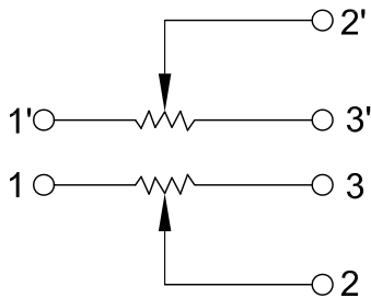
接线图 Circuit explanation
