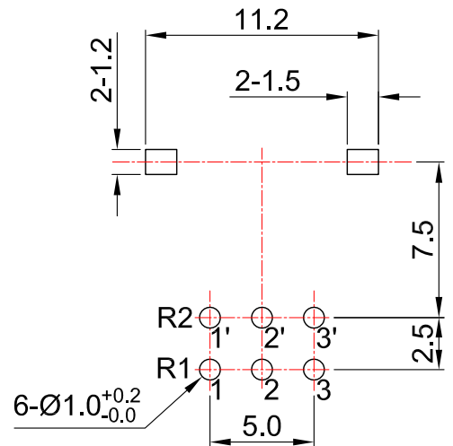
安装孔位置图 P.C.B. mounting hole detail
